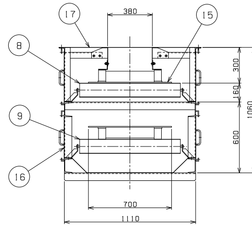
断面 A-A (S=1:15)
